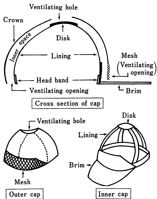
図2 改良型防暑帽の断面図と構造
